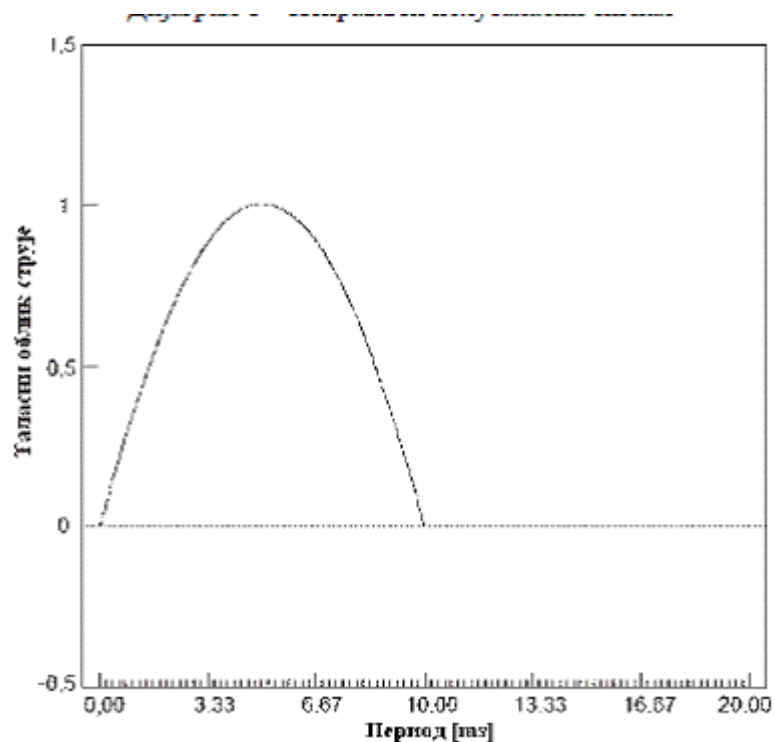
Dijagram 1 - Ispravljen polutalasni signal
