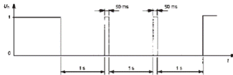
Dijagram 2 - Prekidi električnog napona \Delta U = 100\%
