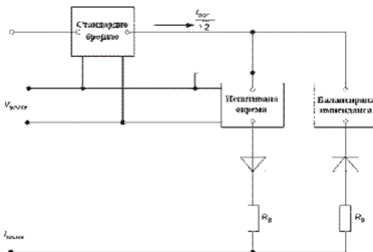
Slika 2 - Kolo za ispitivanje uticaja komponente jednosmerne električne struje
